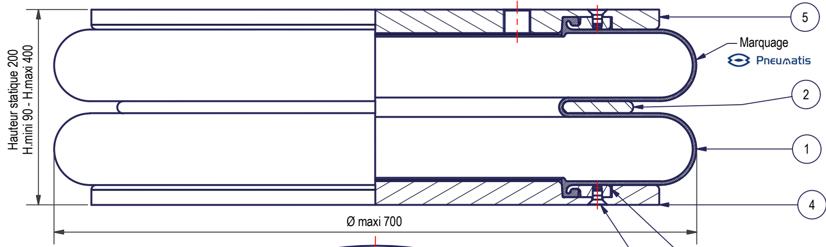
Coupe A-A
