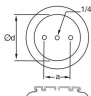
Type A à flasques
