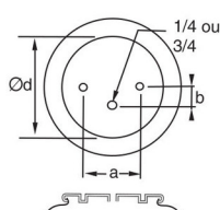
Type C à flasques
