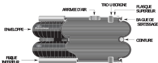
A flasques avec bague de sertissage Type F
