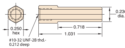
11675-08 1/4" OD Tube
