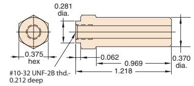
11675-12 3/8" OD Tube
